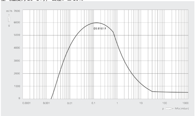
抽气速率
